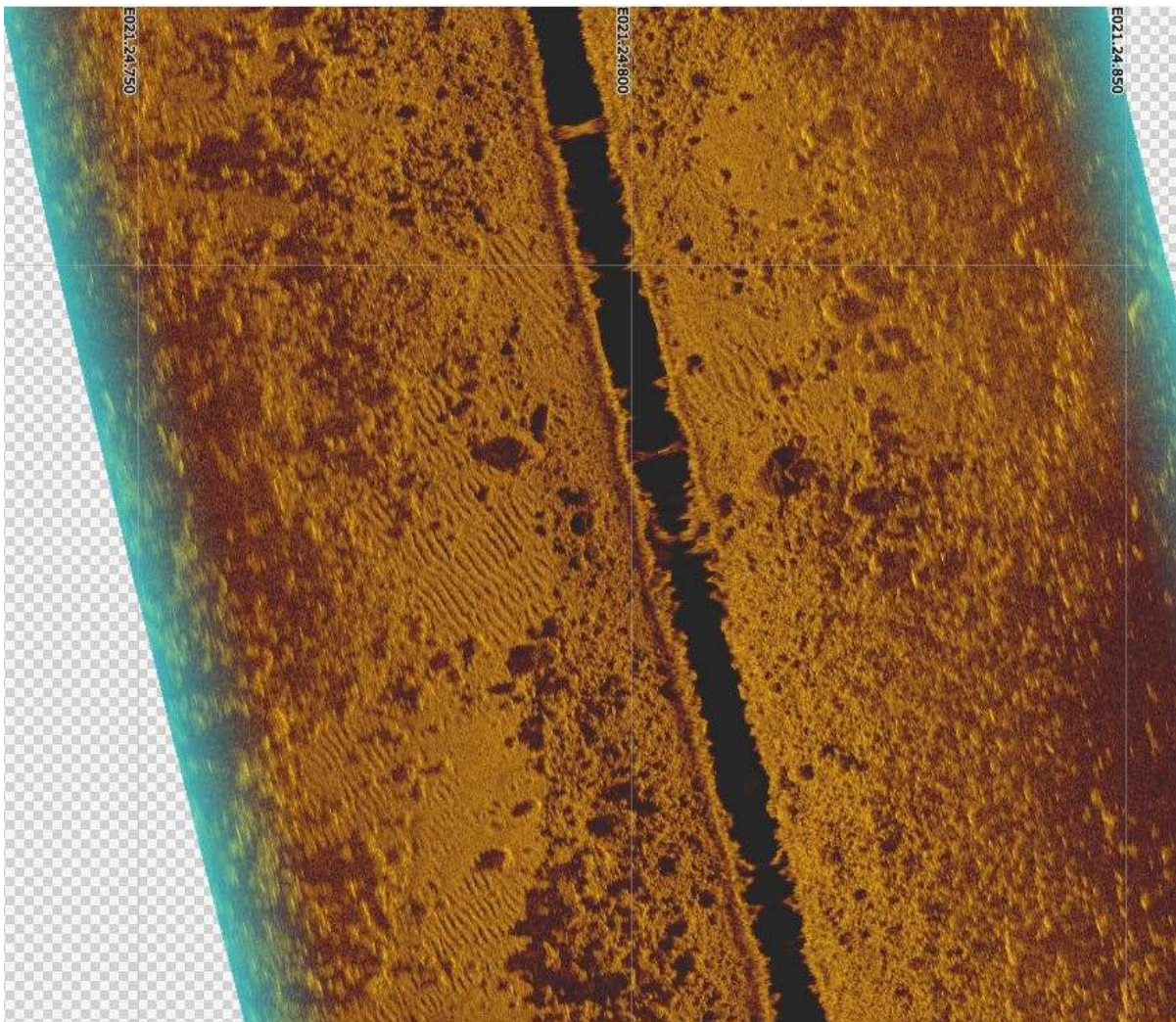
Kuva 9. Tyypillinen pohjan koostumus, jossa näkyy hiekkaa, soraa ja muutamia suurempia kivilohkareita. Hiekkaan on muodostunut aaltokuviota.
