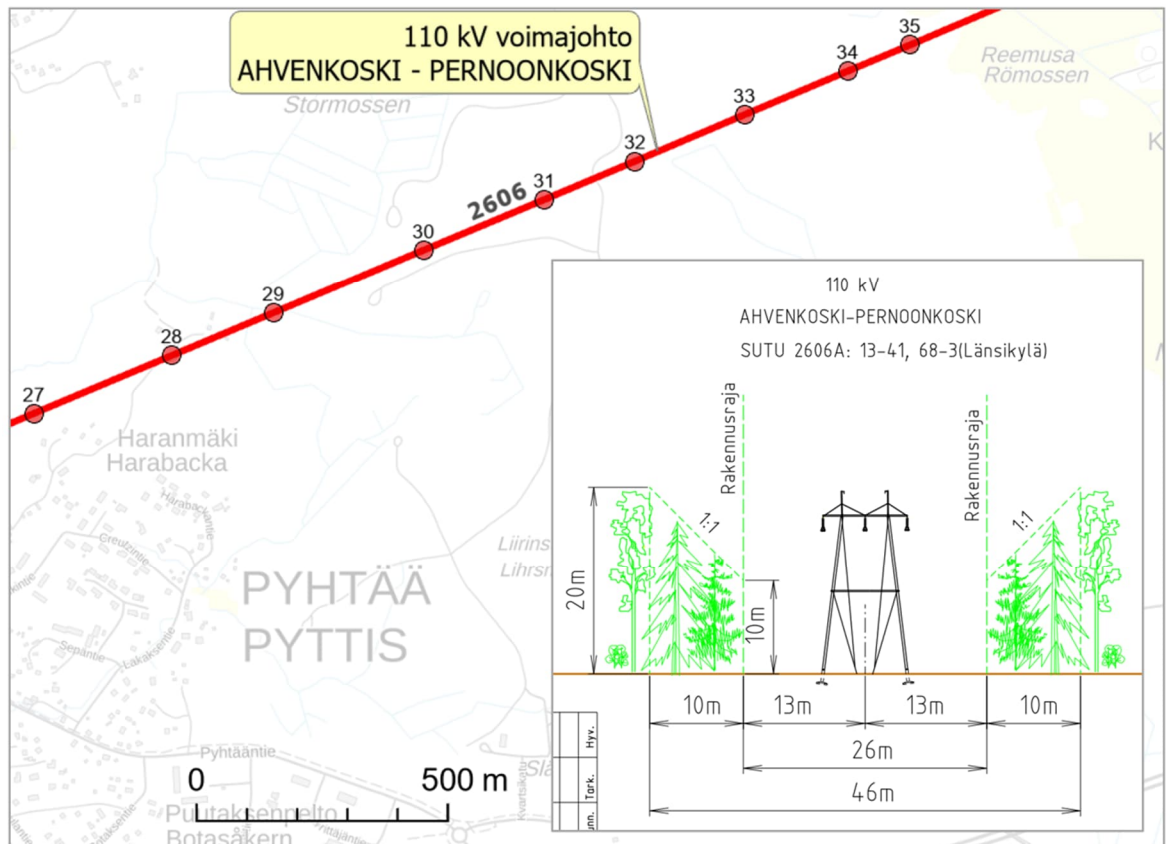
Kuva 1. Fingridin voimajohto.
